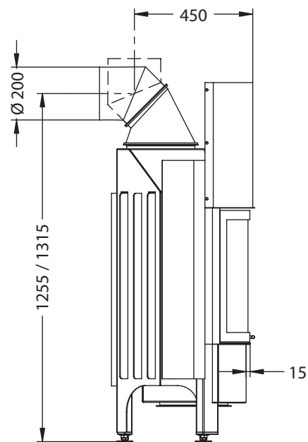
Seitenansicht M~1:20
