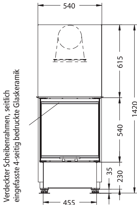
Vorderansicht M~1:20
